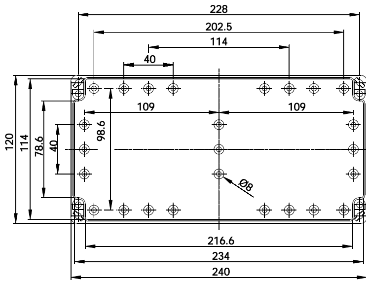
Unterteil bottom / base part
