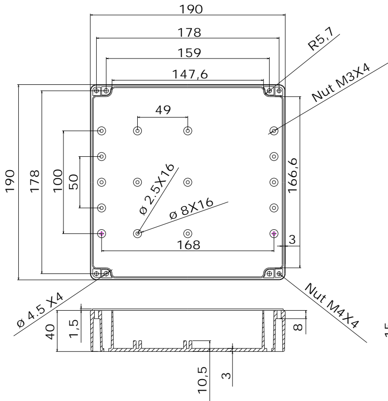
Unterteil bottom / base part
