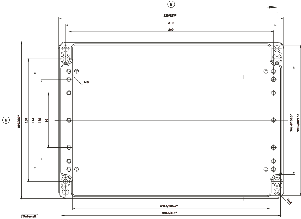
Unterteil
