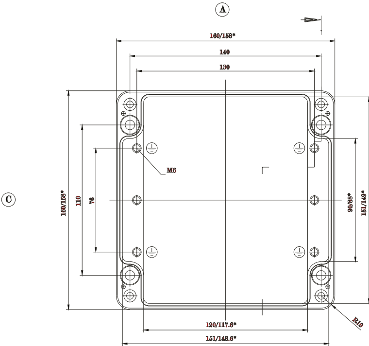
Unterteil
